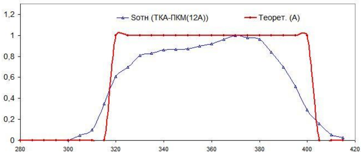
Рис.1 Относительная спектральная чувствительность прибора
