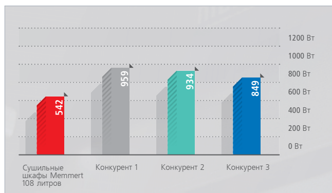
Теплоотдача при 250 °C, воздушная заслонка закрыта
